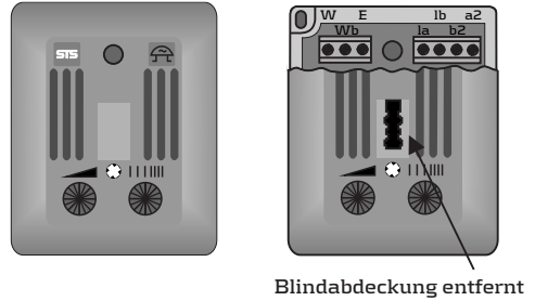
Blindabdeckung entfernt
